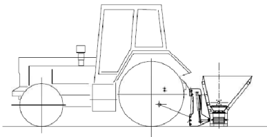
1 - EN REPOSO ENGANCHE EN LAS BARRAS DE ALZAMIENTO
